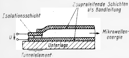
Bild 11. Tunnellelement als Mikrowellengenerator
