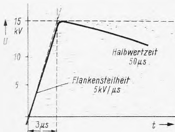
Bild 8. Prüfpulse für die Messung der Ansprechstoßspannung.
