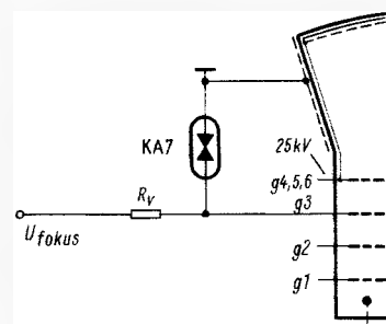
Bild 3. Schutz der Bildröhre durch einen Überspannungsableiter KA 7
