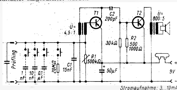
Schaltung eines einfachen Prüfergerätes für Kondensatoren von 100 pF bis 10 \mu F
