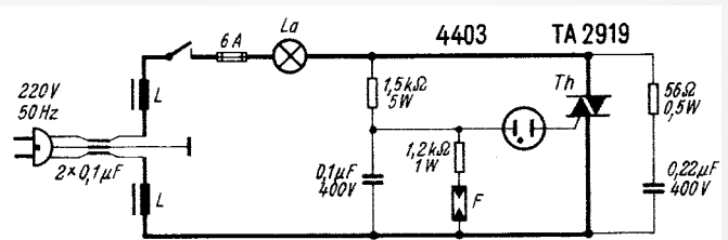
Bild 21. Schaltung zum automatischen Ein- und Ausschalten von Lampen in Abhängigkeit von der Tageshelligkeit mit Hilfe eines Fotowiderstandes F
