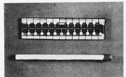
Bild 3b. Kreuzkryotron auf einer 1 cm x 4 cm großen Glasplatte. Am Rand sind die eingebrannten Silberkontakte zu erkennen, an denen die Leitungen festgelötet werden (Werkaufnahmen: Siemens)
