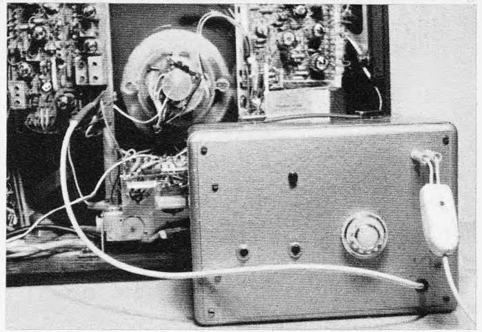
Bild 3.04-5. Unabhängiger VHF-Konverter
