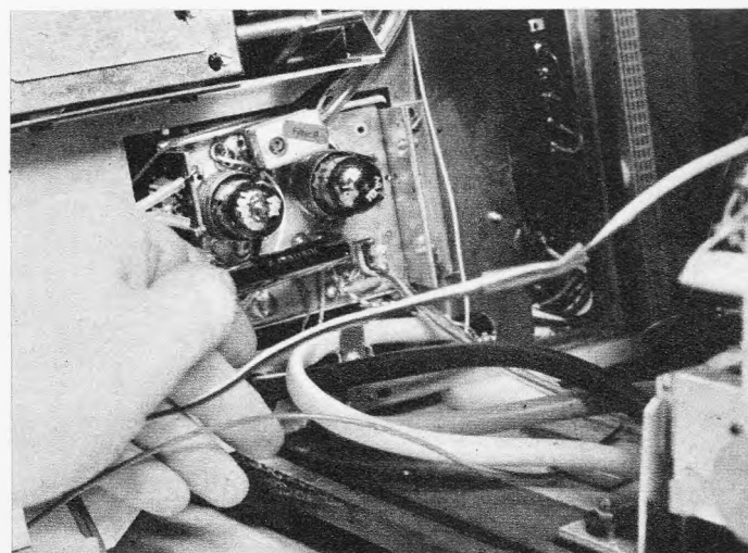
Bild 3.04-3. Anlegen eines Sperrschringers (Minitest II) an den VHF-Kanalschalter
