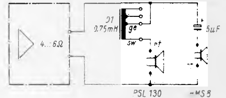
Bild 1. Schaltung der Lautsprecher in der Box
