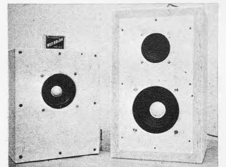
Bild 2. Laboraufbau der Box; links daneben eine 3,6-Liter-Box mit Doppelkonuslautsprecher
