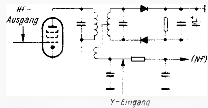
Bild 17. Prinzip des Zf-Abgleichs in UKW-Rundfunk- und Fernseh-ton-Empfangsteilen. Der Hf-Ausgang des Wobblers liegt über 60 \Omega/0,1 \mu\text{F} am Gitter der letzten Zf-Stufe
