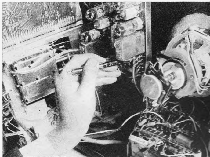
Bild 3.04-2. Anlegen eines Sperrschringers (Minitest II) an den Zf-Verstärker
