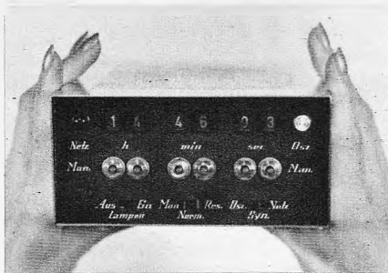
Applikationsmuster einer Digital-Uhr, aufgebaut aus 37 monolithischen Schaltungen (Werkaufnahme: SGS-Fairchild)
