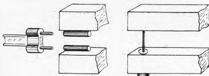
Bild 2. Steckverbindungen für logarithmisch-periodische Antennen (links) und zum Zusammen-schalten nach dem Vorschlag (rechts)
