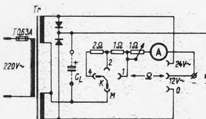
Bild 1. Die Schaltung des vielseitig verwendbaren Ladegerätes
