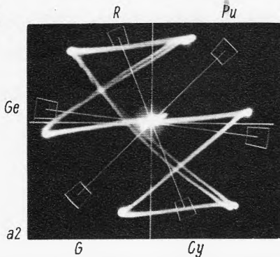
Bild 92. Zeigerdiagramm einer Treppenbalkenfolge sowie (R' - Y') -Farbdifferenzsignale bei falscher (a) und bei richtiger Phasenlage (b) der Pal-Schaltimpulse
