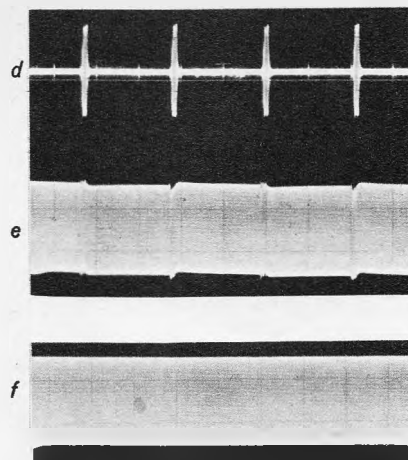
Bild 88. a = Burst-Schwingungszug, b = 4,43-MHz-Referenzträgeroszillator-Schwingungszug, c = 4,43-MHz-Referenzträger-Schwingungszug mit Verzerrungen bei falscher Amplitudeneinstellung, d = Burst-Schwingungen, e = Oszillogramm der 4,43-MHz-Referenzträgeroszillator-Schwingung bei vorhandenem Burst. Die Amplitudenänderungen im Zeitpunkt des Burstes kommen durch die periodische 90°-Phasenänderung (Wobbelburst) zustande, f = Oszillogramm der 4,43-MHz-Referenzträgeroszillatorschwingung bei ausgefallenem Burst oder Ausfall des Nachstimmverstärkertransistors T 406
