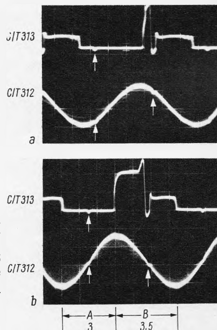
Bild 90. a = Pal-Kennimpuls sowie Schwingung des 7,8-kHz-Pal-Kennimpulsverstärkers bei falschem Abgleich des Kreises L 312 und falscher Einstellung von R 368 (Triggerimpulseeinsatz), b = bei richtiger Einstellung
