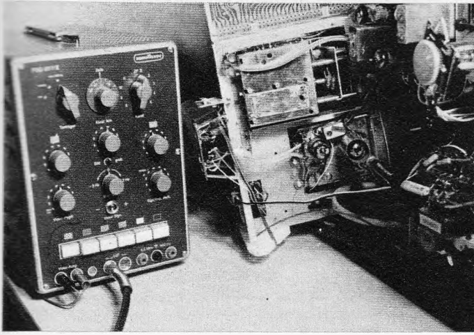
Bild 3.04-4. Anlegen des Zf-Signales aus dem Bildmuster-generator über eine Aufblaskappe in den Kanalschalter
