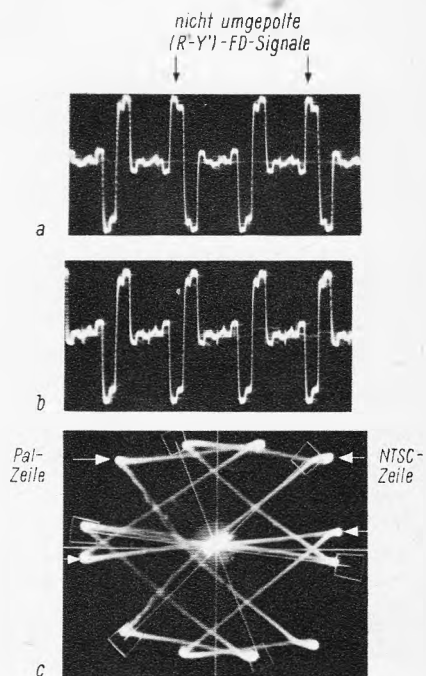
Bild 92. Zeigerdiagramm einer Treppenbalkenfolge sowie (R' - Y') -Farbdifferenzsignale bei falscher (a) und bei richtiger Phasenlage (b) der Pal-Schaltimpulse
