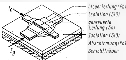
Bild 3a. Kreuzkryotron
