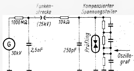
Bild 7. Messung der Ansprechstoßspannung U_{as} .
