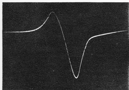
Bild 18. Schirmbild einer Diskriminatorekurve
