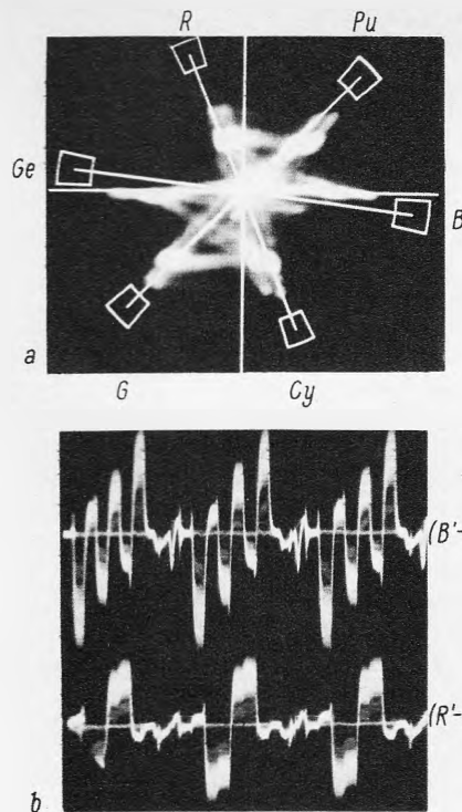
Bild 86. Zeigerdiagramm (a) sowie FD-Signale (b) bei Verstimmung des Referenzträgeroszillators oder des Farbdemodulatorkreises, wenn die Oszillatorfrequenz in der Nähe der Grenzen des Fangbereichs liegt. Referenzträgeroszillator wird noch synchronisiert, das Farbbild „flackert“ jedoch bereits leicht
