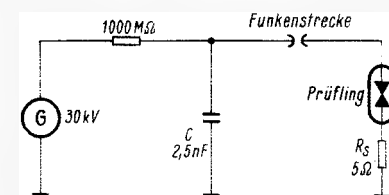
Bild 5. Lebensdauerprüfung von Überspannungsableitern des Typs KA 7
