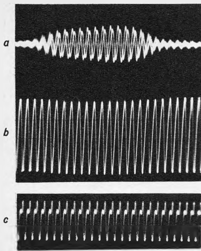
Bild 88. a = Burst-Schwingungszug, b = 4,43-MHz-Referenzträgeroszillator-Schwingungszug, c = 4,43-MHz-Referenzträger-Schwingungszug mit Verzerrungen bei falscher Amplitudeneinstellung, d = Burst-Schwingungen, e = Oszillogramm der 4,43-MHz-Referenzträgeroszillator-Schwingung bei vorhandenem Burst. Die Amplitudenänderungen im Zeitpunkt des Burstes kommen durch die periodische 90°-Phasenänderung (Wobbelburst) zustande, f = Oszillogramm der 4,43-MHz-Referenzträgeroszillatorschwingung bei ausgefallenem Burst oder Ausfall des Nachstimmverstärkertransistors T 406
