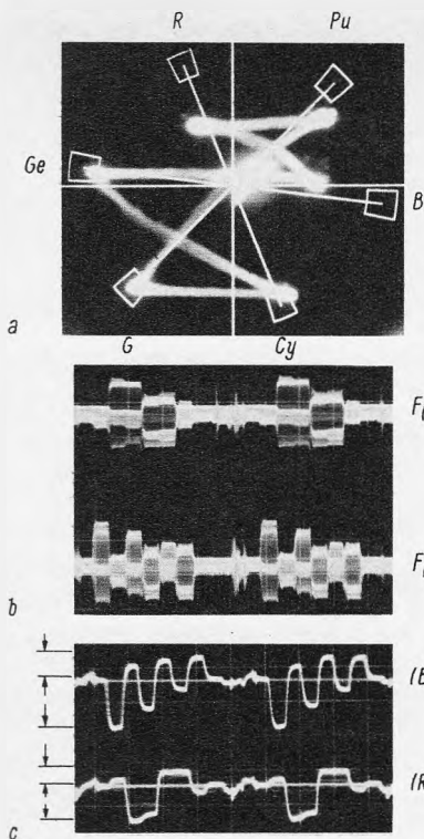
Bild 85. Zeigerdiagramm (a), getragene FD-Signale (b) im Farbdemodulatorfilter F 16 (vgl. Bild 38 und 79) sowie FD-Signale (c) bei Verstimmung des Referenzträgeroszillatorkreises L 441, des Referenzträgeroszillators mit R 442 im Filter F 15 oder des Farbdemodulatorkreises L 451/L 452-L 453 im Filter F 16 (vgl. Bild 80 und die Oszillogramme in Bild 79)
