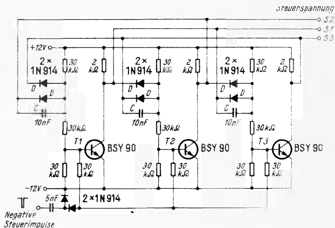
Bild 2. Addition von steuernden Vorspannungen
