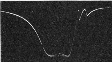
Bild 23. Durchlaßkurve mit eingeblendeter Frequenzmarke
