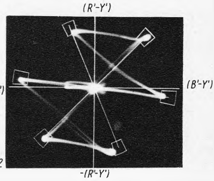
Bild 92. Zeigerdiagramm einer Treppenbalkenfolge sowie (R' - Y') -Farbdifferenzsignale bei falscher (a) und bei richtiger Phasenlage (b) der Pal-Schaltimpulse
